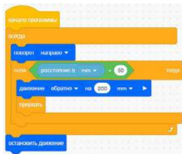
Рис. 57. Пример программы
